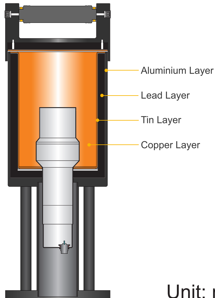
SECTION A-A
