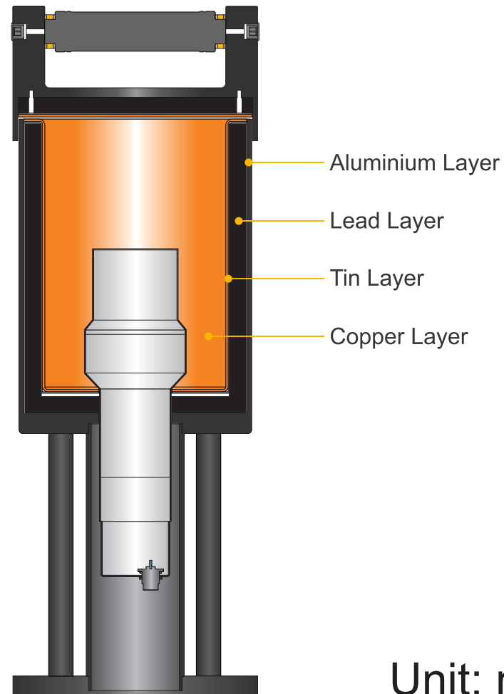
SECTION A-A
